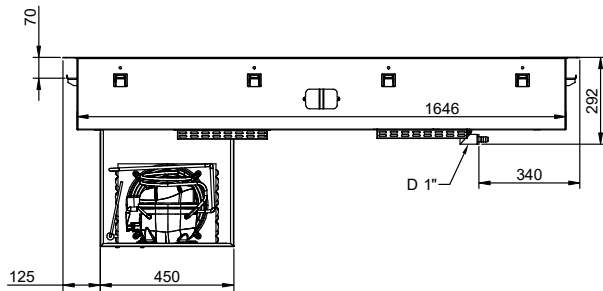
Zij aanzicht
